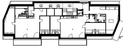
Regelgeschoss Dachgeschoss
