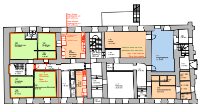
Sicherheitspläne und Nutzungsstudie Provisorische Residenz
