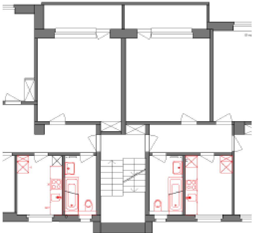
Wabersackerstrasse 85 Liebefeld Sanierung Wohngebäude, verschiedene Etappen
