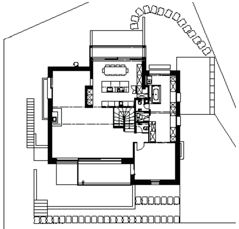
Erdgeschossplan
