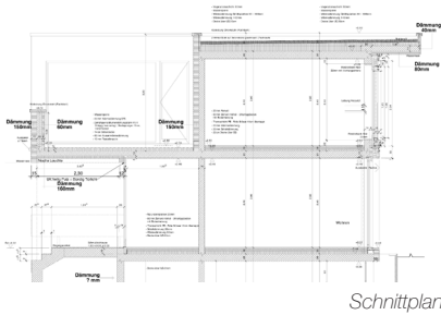
Schnittplan
