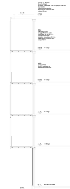
Coupe constructive Bâtiment
