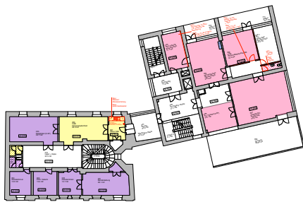
Sicherheitspläne und Nutzungsstudie Provisorische Kanzlei
