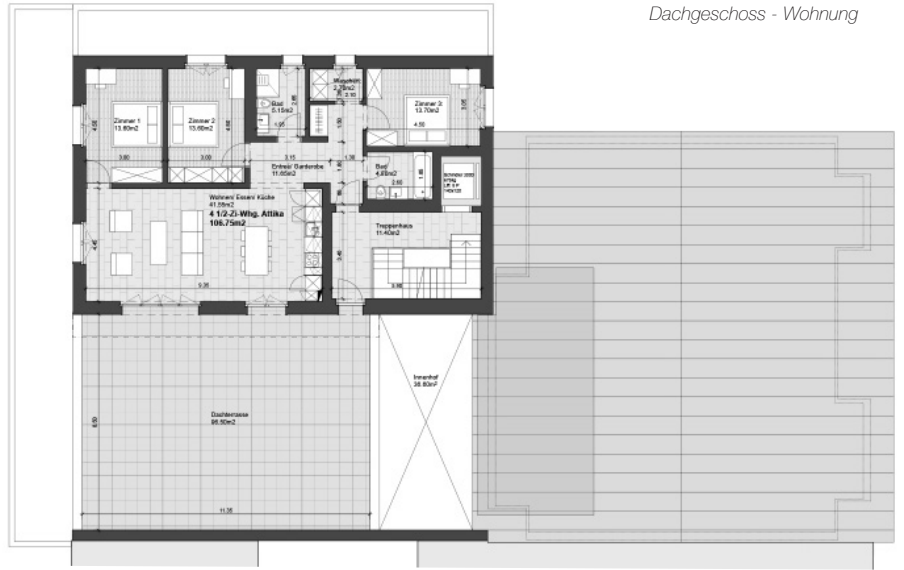
Erweiterung Güterstrasse 22 Bern Innenbereich
